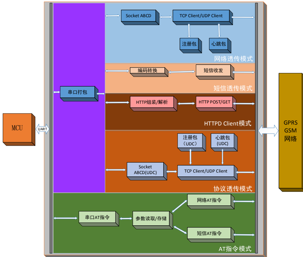
图 1 功能框图
