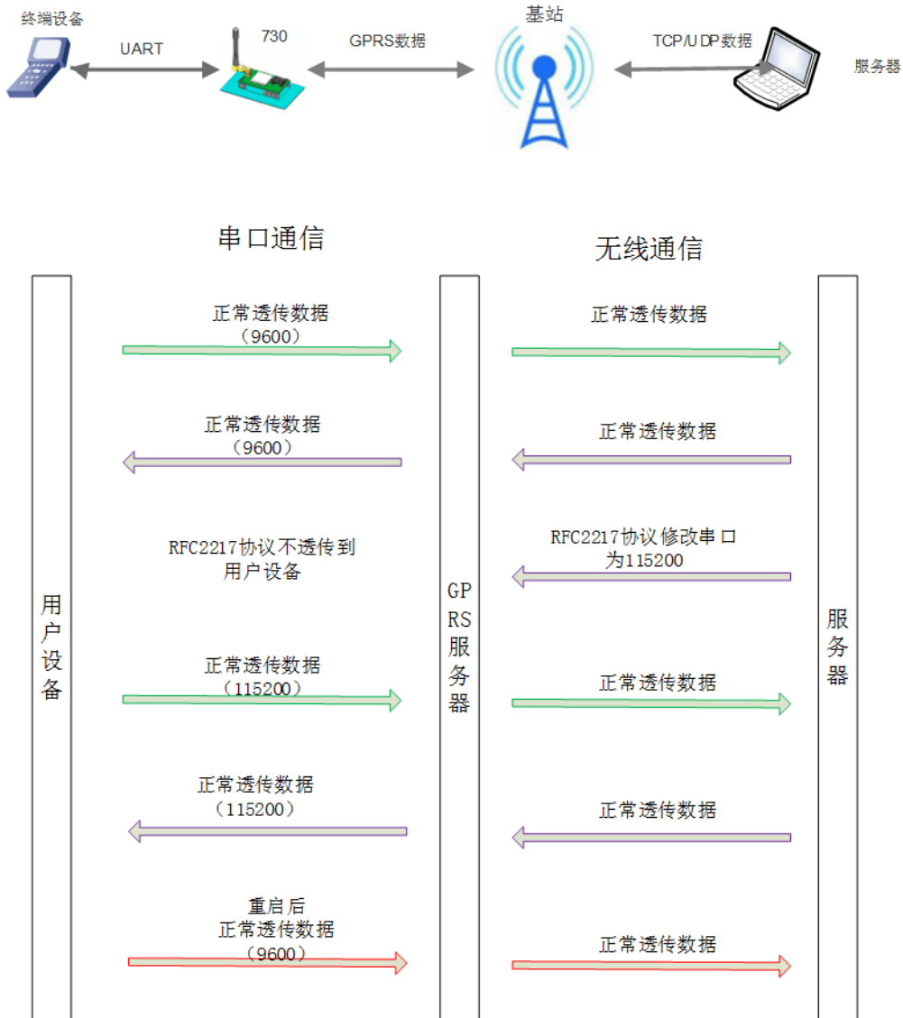
图 12 类 RFC2217 功能逻辑示意图
