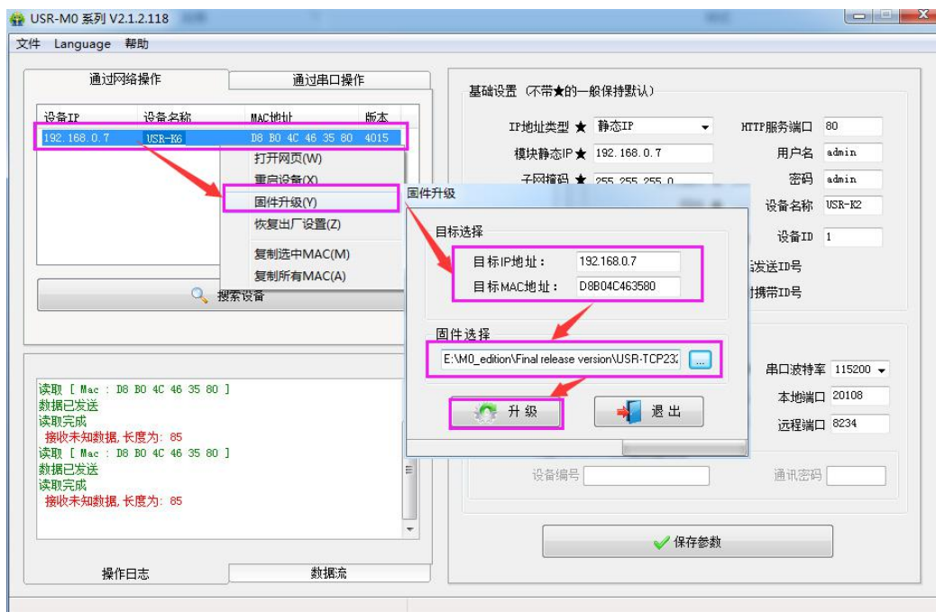
图 5. 选择固件
