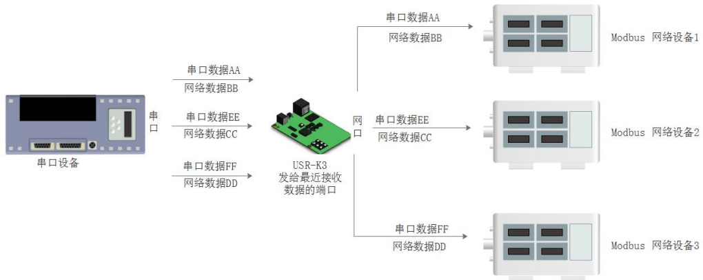
图 46 Modbus TCP
