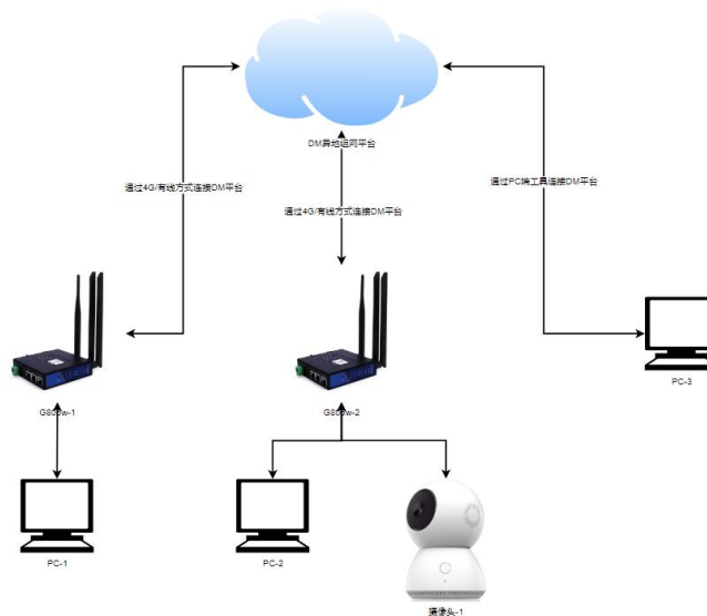
图 10 组网拓扑
