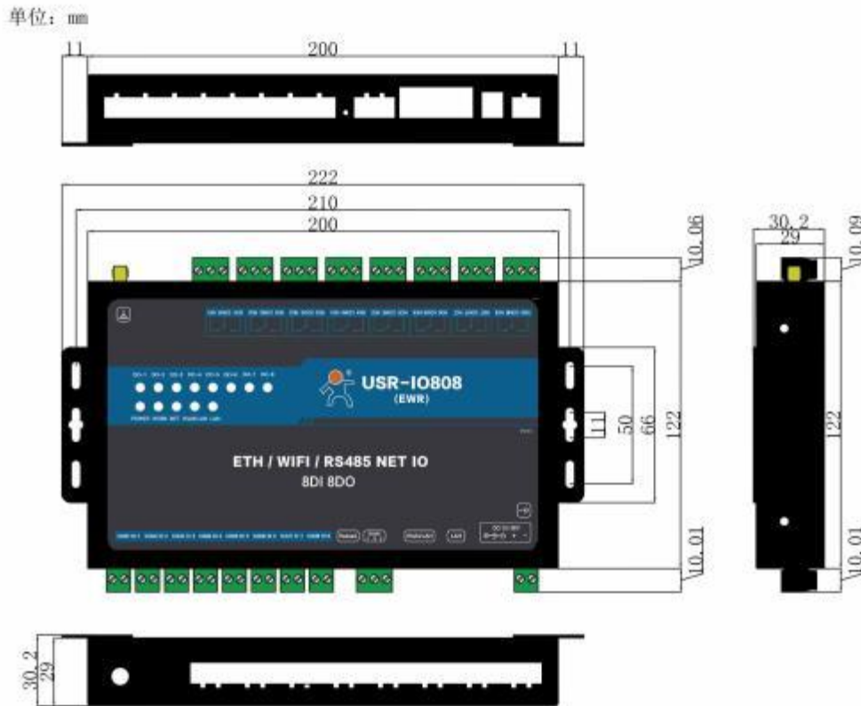
IO808-EWR外观尺寸图
