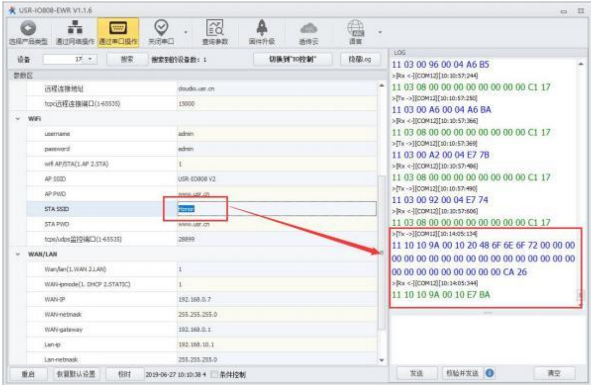
图 14 修改参数
