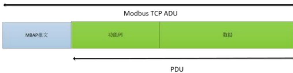
图 41 Modbus TCP 帧
