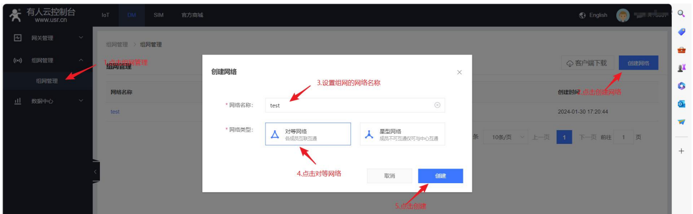
图 7 创建网络
