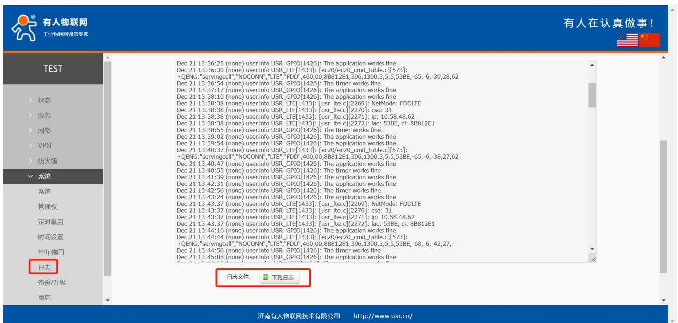
图 84 导出日志
