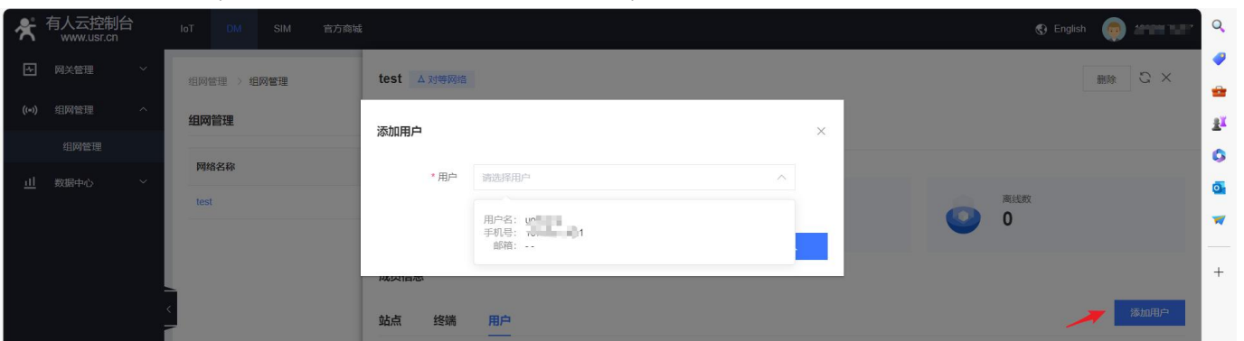
图 11 添加用户
