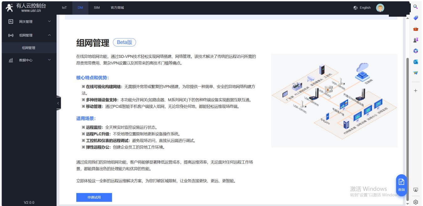
图 6 组网申请
