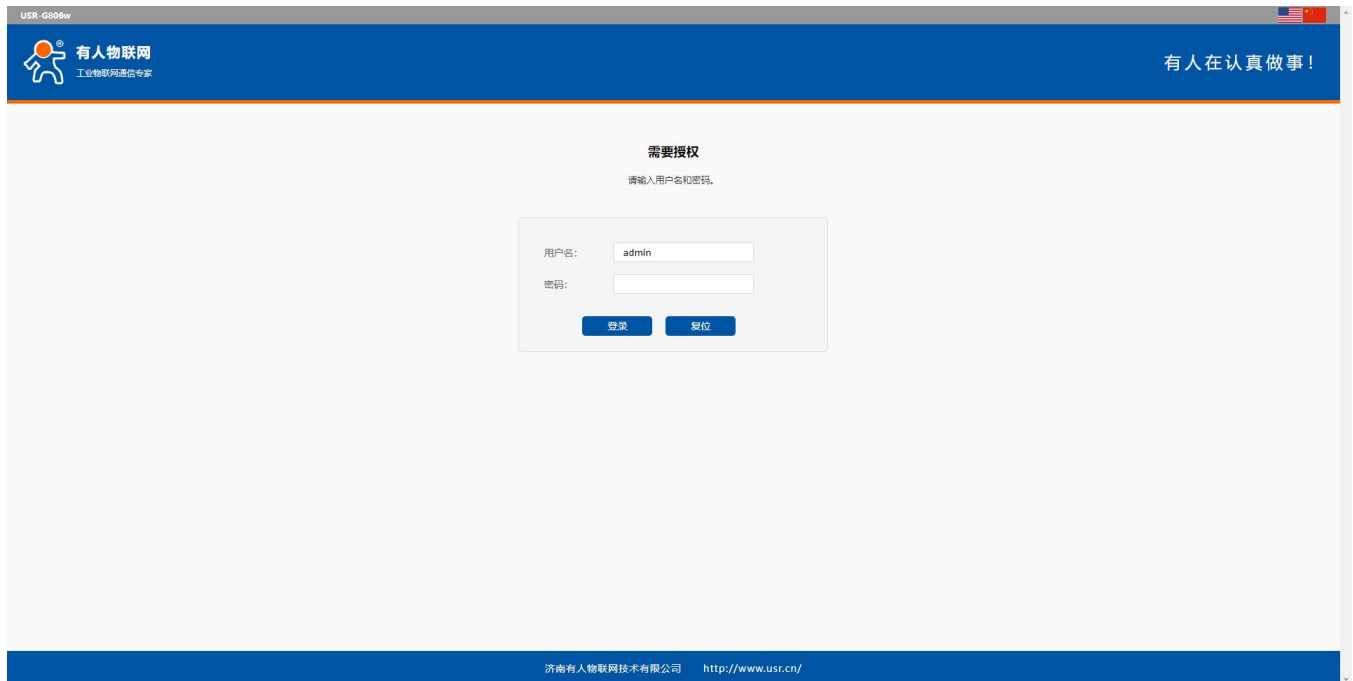
图 2 首页页面
