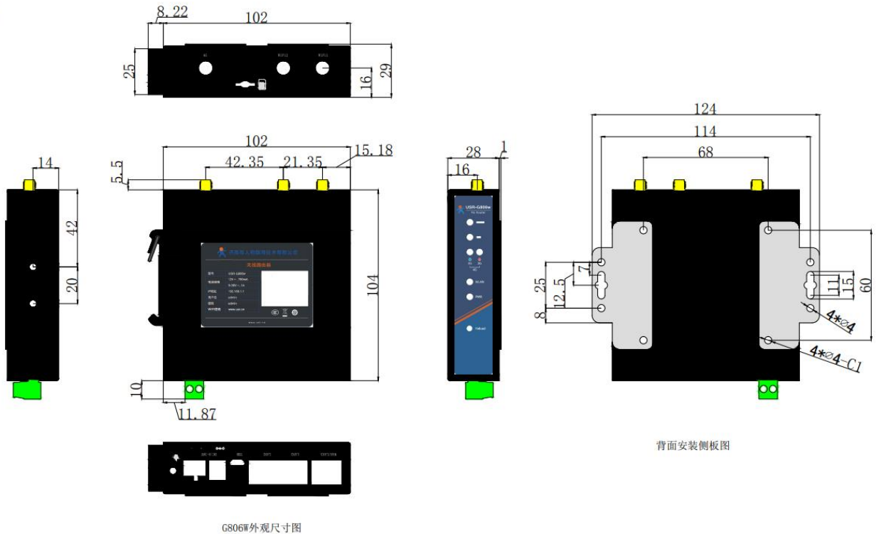
图 1 USR-G806w 尺寸图
